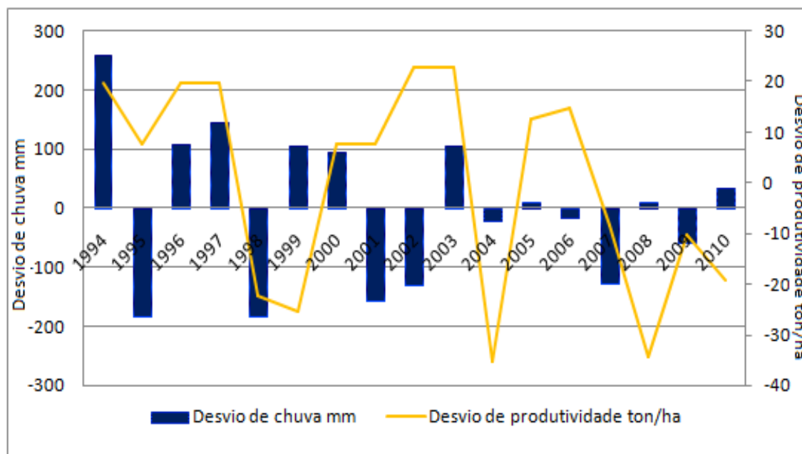
Figura 04- Desvios de chuva e produtividade do milho no município de Feira de Santana (Bahia) no período de 1994 a 2010. Fonte dos dados: Estação Climatológica/UEFS (2012).
