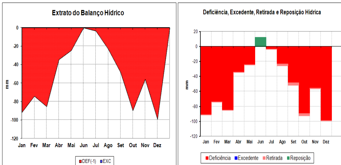
Figuras 02 e 03 - Gráfico do Balanço Hídrico Climático (Thornthwaite e Mather, 1955) no município de Feira de Santana (Bahia) de 1994 a 2010.
